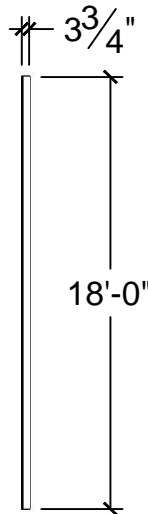
3 SIDE VIEW Scale: 1/8" = 1'-0"
