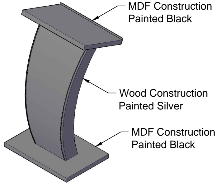
5 ISO VIEW Scale: 5/8" = 1'-0"
