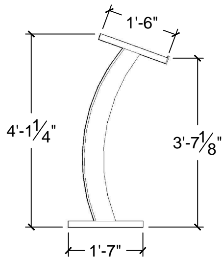
3 SIDE VIEW Scale: 1/2" = 1'-0"
