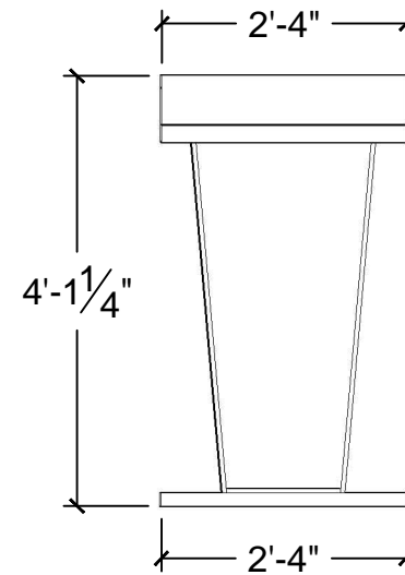
4 BACK VIEW Scale: 1/2" = 1'-0"
